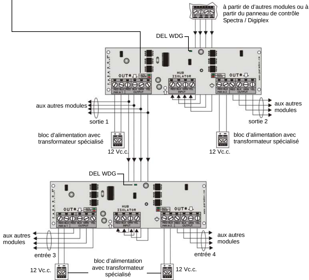
Figure 2 : Raccordement du APR3-HUB2
