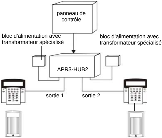
Figure 1 : Vue d'ensemble du APR3-HUB2
