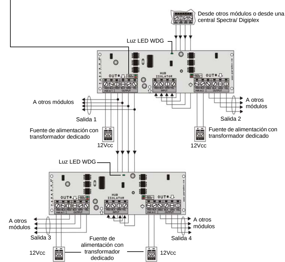
Figure 2 : Conexión del APR3-HUB2
